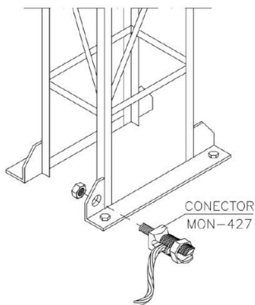
CONEXÃO MASSA METÁLICA
