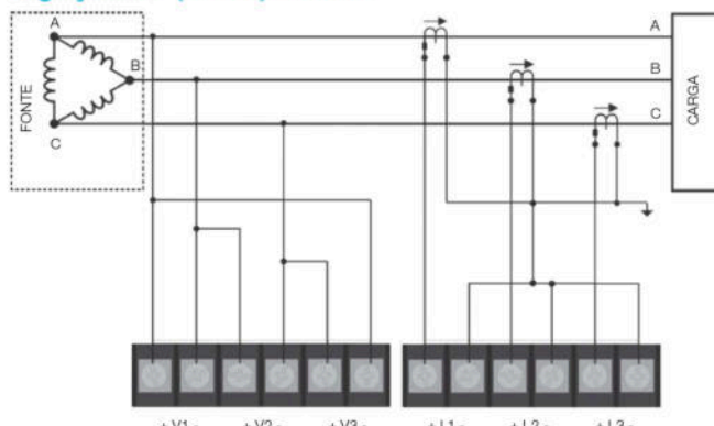
3P3W-3V3C - Trifásico 3 Fios, Delta, Conexão Direta, 3 TC
