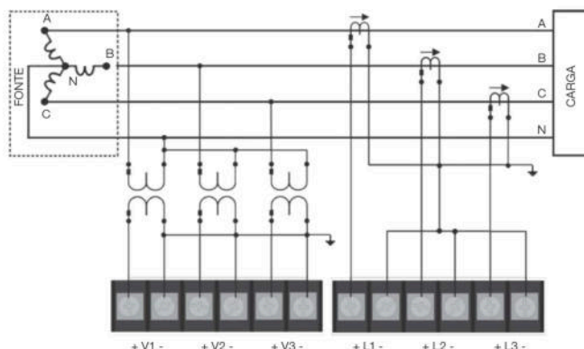
3P4W-3V3C - Trifásico 4 Fios, Estrela, Conexão 3 TP, 3 TC
