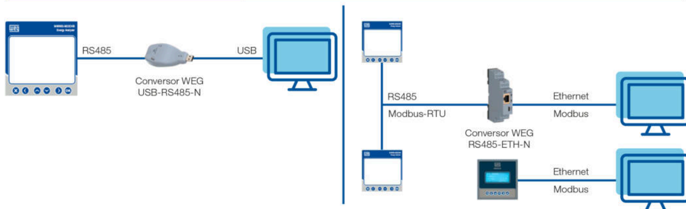
Parametrização do MMW utilizando o conversor USB/RS485 ou o conversor RS485/ETH-N ou direto Ethernet.
