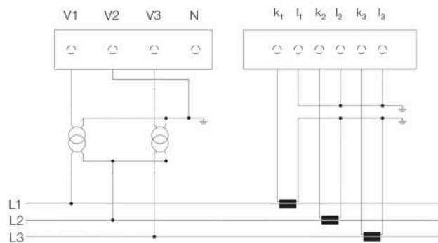
Medição com 2 TP e 3 TCs
