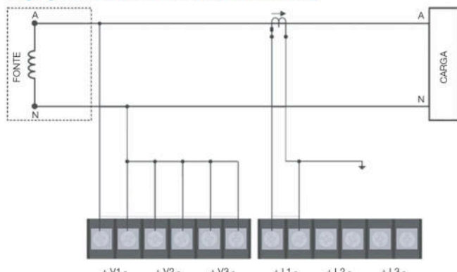
1P2W-1V1C - Monofásico (LN)
