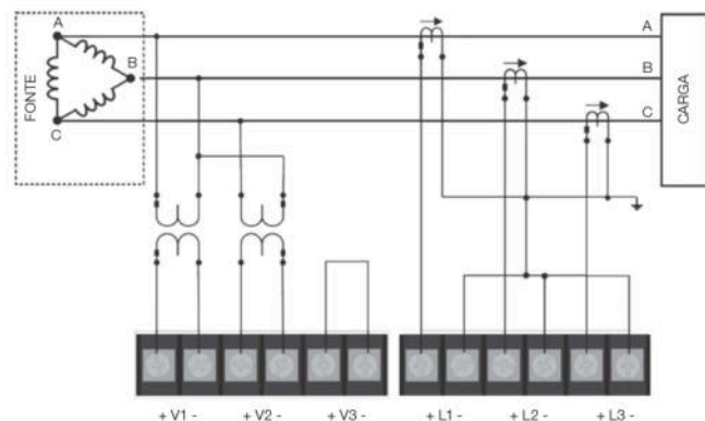
3P3W-2V3C - Trifásico 3 Fios, Delta, Conexão 2 TP, 3 TC
