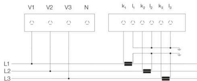
Medição direta de tensão e corrente com 3 TCs
