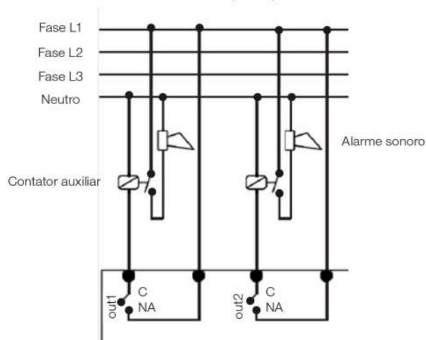
Sugestão de ligação conexão dos relés de saídas de alarme OUT1 e OUT2 (alarme)
