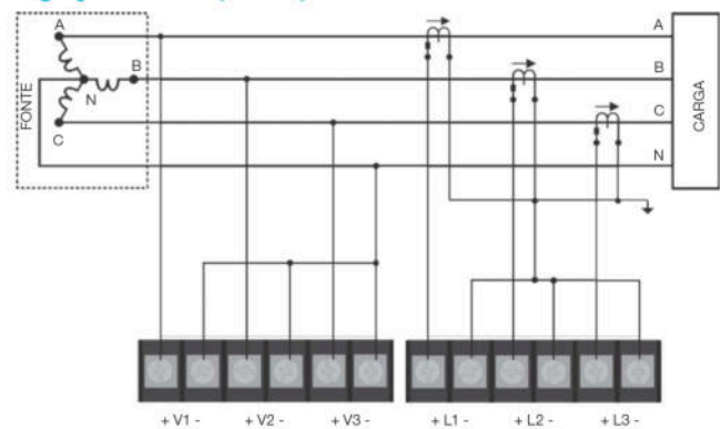
3P4W-3V3C - Trifásico 4 Fios, Estrela, Conexão Direta, 3 TC
