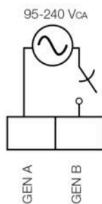
Conexão das entradas GEN
