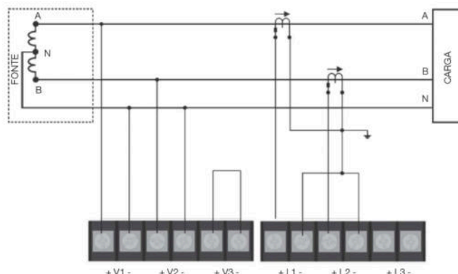
2P3W-2V2C - Bifásico (LL+N)
