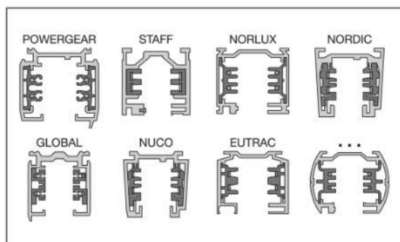
Calhas Compatíveis
