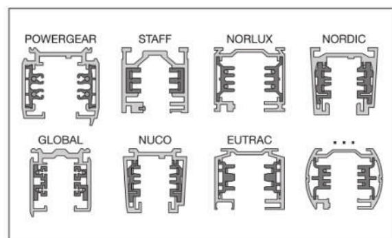
Calhas compatíveis
