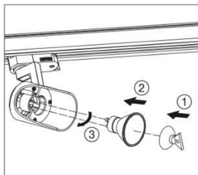
Instalação de uma lâmpada (não incluída)
