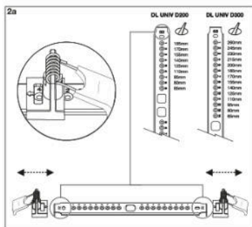
Molas ajustáveis
