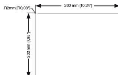
Dimensões do rasgo do painel
