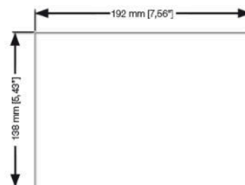
Dimensões do rasgo do painel
